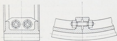
Abb. 1902. Kranzverbindung.
