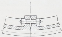
Abb. 1902. Kranzverbindung.
