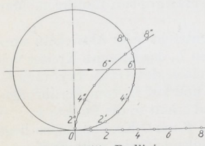
Abb. 1845. Radlinie.
