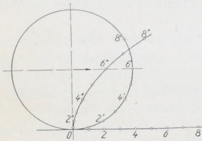
Abb. 1845. Radlinie.
