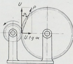
Abb. 1836. Unzweckmäßige Aufnahme des Radialdrucks an Zahngetrieben.
