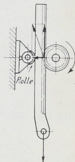
Abb. 1837. Aufnahme des Radialdrucks an einer Zahnstange.
