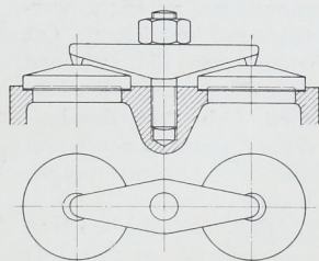
Abb. 1781 und 1782. Bügelverschlüsse.
