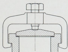
Abb. 1781 und 1782. Bügelverschlüsse.
