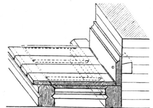
Amerikanischer kalfatertes Fußboden 43) .
