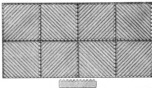
Neuzeitliche Tonfliesen.
