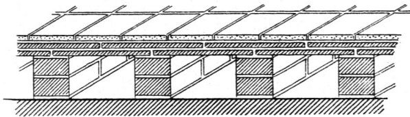
Kanäle zum Erwärmen des Fußbodens.
