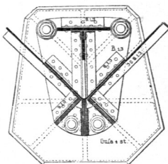
Auflegerplatte.
