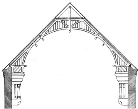
Satteldachbinder.
