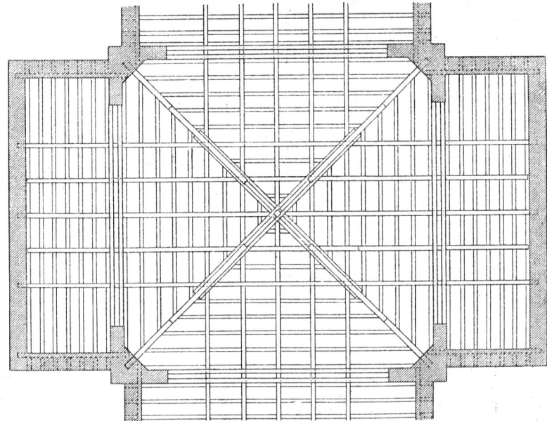
Grundriss.
