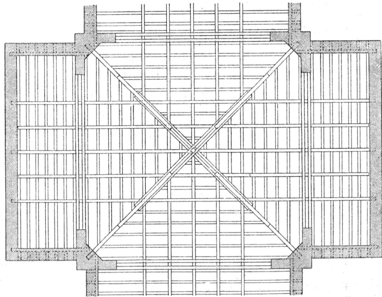
Grundriss.
