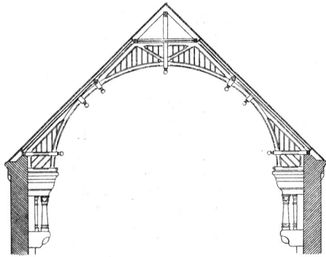
Satteldachbinder.
