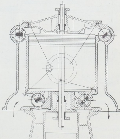
Abb. 1744. Zylinder für stehende Maschine nach Doerfler.
