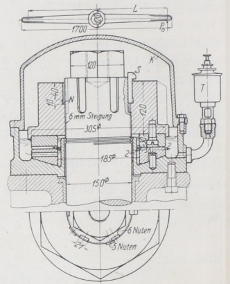
Abb. 1588. Turbinenstützlager für 5000 kg Druck. M. 1: 10 und 1: 50.
