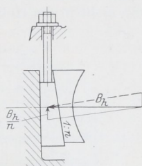
Abb. 1585. Zur Berechnung der Keilschrauben am Lager, Abb. 1583.
