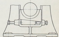
Abb. 1514. Lager mit Keilnachstellung.
