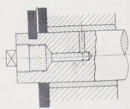
Abb. 1480. Staufferbüchse in einer Achse.
