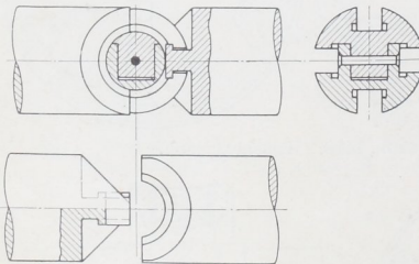
Abb. 1422. Kreuzgelenkkupplung.
