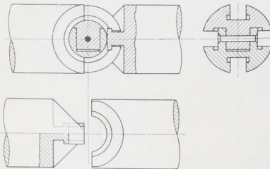
Abb. 1422. Kreuzgelenkkupplung.
