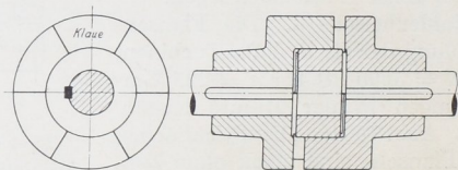
Abb. 1408. Klauenkupplung mit Zentrierung.
