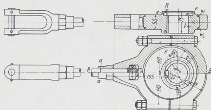
Abb. 1390. Genormtes Exzenter für Ventilsteuerungen. M. 1:10.
