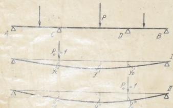
Abb. 1346. Zur Berechnung mehrfach statisch unbestimmter Wellen.
