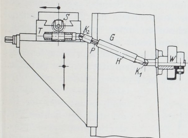
Abb. 1290. Antrieb eines Frässlittens durch eine Gelenkwelle.
