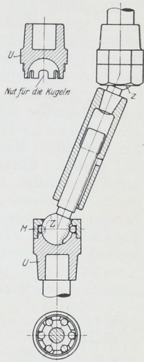
Abb. 1291. Gelenkwelle von C. Klingelhöffer, Grevenbroich.
