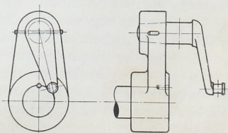
Abb. 1294. Gegenkurbel.
