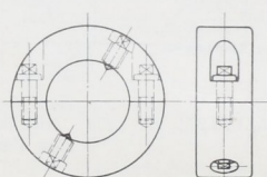
Abb. 1277. Geteilter Stelling.
