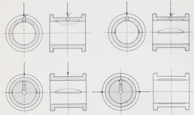
Abb. 1230 bis 1233. Schmierung von Kreuzkopfpapfen.
