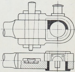
Abb. 1222. Veraltete Stangenkopfform.
