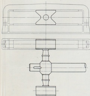
Abb. 1184. Veraltete Form des Kreuzkopfes.
