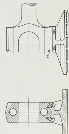
Abb. 1186. Abänderung des Kreuzkopfes Abb. 1185.
