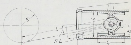
Abb. 1165. Ermittlung der Kreuzkopfhöhe.
