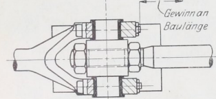
Abb. 1159 und 1160. Hauptformen der Kreuzköpfe: gabelförmige und geschlossene Bauart.
