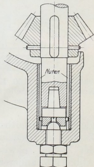
Abb. 1157. Stützlager einer Reglerspindel.
