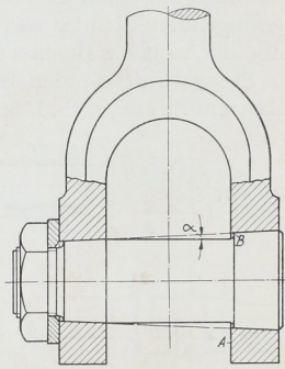
Abb. 1152. Gabelzapfen mit kegeligem durchlaufendem Sitz.
