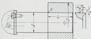
Abb. 1139. Falsche Anordnungen von Bunden.
