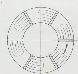
Abb. 1133. Ausbildung keiliger Schmierschichten an einem Stützlager.
