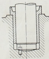
Abb. 1083. Stütz- oder Spurzapfen mit Halslager.
