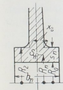
Abb. 2288. Bezeichnungen an der Nabe von Scheiben.
