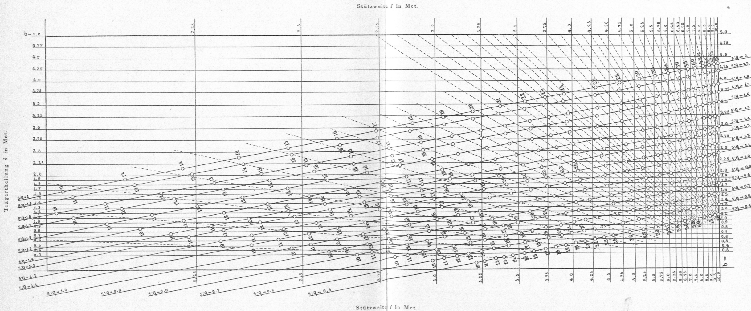
Zeichnerische Darstellung der Normal-I-Eifen für die Untersuchung ihrer Tragfähigkeit unter lothrechter Belastung.
