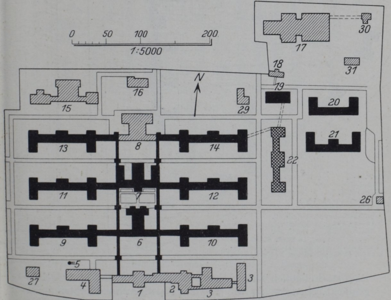
Abb. 234. München-Schwabing, städt. Krankenhaus für 1300 Betten. 1 Hauptgebäude. 2 Kapelle. 3 Schwesternhaus. 4 Verwaltung u. Apotheke. 6 Operationshaus. 7 Badehaus. 8 Kochküche. 9—10 äußere Abteilung. 11—14 innere Abteilung. 15 Waschhaus u. Desinfektion. 16 Gärtnerei. 17 Kessel- u. Maschinenhaus. 18 Tierstall. 19 Pathol. Institut. 20, 21, Absonderungshaus. 22 Haut- und Geschlechtskranke. 27 Direktorwohnhaus. 29 Zentralregulierhaus. 30 Kohlenkipperhaus. 31 Dienstwohngebäude.
