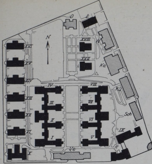
Abb. 233. Berlin-Charlottenburg, städt. Krankenhaus „Westend“, 662, jetzt 1000 Betten. I—IV Äußere Abteil. V bis VIII Innere Abteil. IX Einzelbetten-Haus. X Frauenabteilung. XI bis XVI Absonderungshäuser. XVII—XVIII Leichtkrankenhaus. Ve Verwaltungsgebäude. Sch Schwesternhaus. Kü Kesselhaus. W Waschküche. L Leichenhaus. D Desinfektionshaus. R Röntgenhaus.
