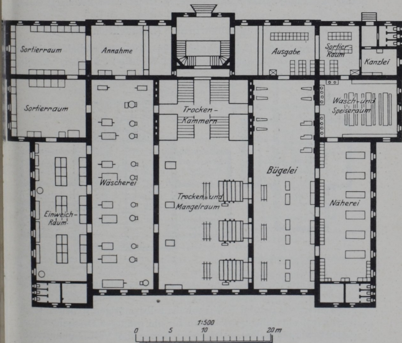
Abb. 193. Wien, Landes-Heil- und Pflegeanstalt „Am Steinhof“ für 3000 Betten, Waschhaus.
