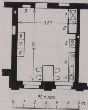
Abb. 23. Mannheim. Städt. Krankenhaus. Teeküche. 1 Speisenaufzug. 2 Wärm- u. Küchenschrank. 3 Gaskocher. 4 Spülbecken. 5 Ausguß. 6 Eisschrank. 7 Tisch. 8 Fliegenschrank. 9 Arzneischrank.
