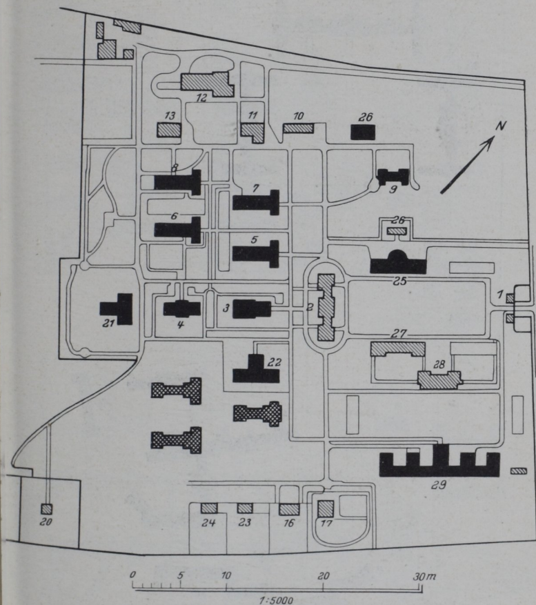
Abb. 230. Zwickau, staatliches Krankstift für 548 Betten. 1 Torhäuser. 2 Verwaltungsgebäude. 3 Operationsgebäude. 4 Privatkanke. 5 bis 8 dreigeschossige Bettenhäuser. 9 Absonderungshaus. 10 Wagenschuppen. 11 Wäscherei. 12 Maschinenhaus. 13 Kochküche. 14 Gärtnerei. 16 und 17 Wohnhäuser. 20 Garten der Schwestern. 21 Badehaus. 22 Dreigeschossiges Bettenhaus. 23 und 24 Wohnhäuser. 25 Pathologisches Institut. 26 Tierställe. 27 und 28 Schwesternhaus. 29 Abteilung für Geburtshilfe und Frauenkrankheiten.
