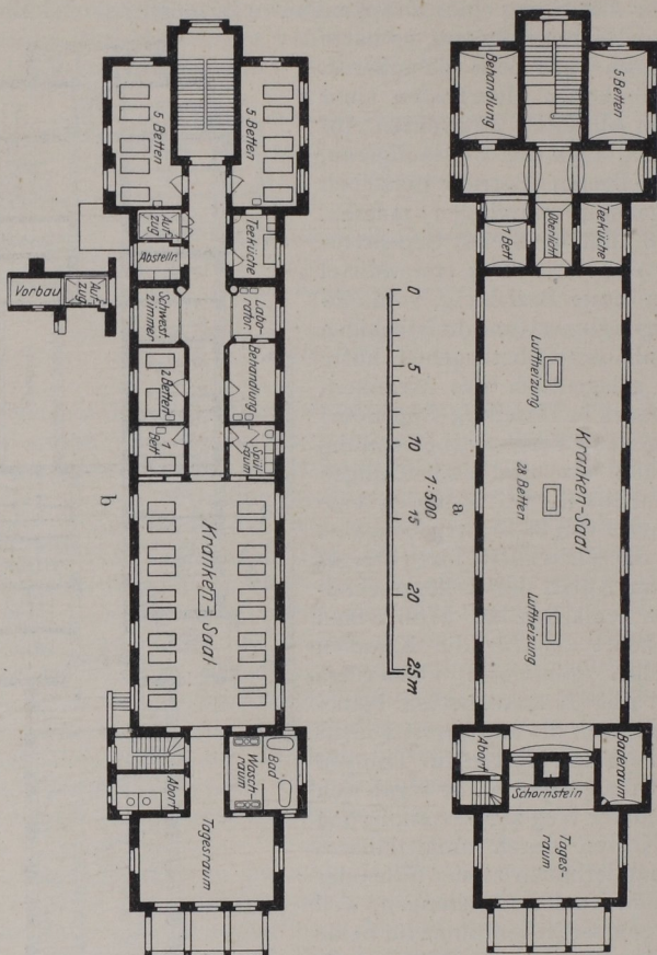
Abb. 111 a u. b. Berlin, städt. Krankenhaus am Friedrichshain, a Bettenhaus 1870—74, b nach dem Umbau 1926—27.
