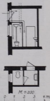
Abb. 28. Einzelabortanlage.
