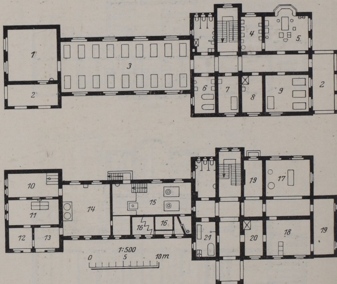
Abb. 206. Petershofen O.-S. Knappschaftskrankenhaus, 80 Betten, Hauptgebäude, Ober- u. Erdgeschoß.
