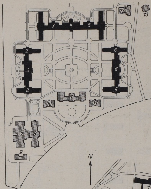
Abb. 231. Wien, Kaiser Jubiläumsspital für 991 Betten. 1 Verwaltungsgebäude. 2, 3, 5 u. 6 Bettenhäuser. 4 Schwesternheim. 7 Kesselhaus. 9 Kraftwagenschuppen. 10 und 11 Ärzte- und Beamtenwohnhaus. 12 Prosektur. 13. Desinfektion.
