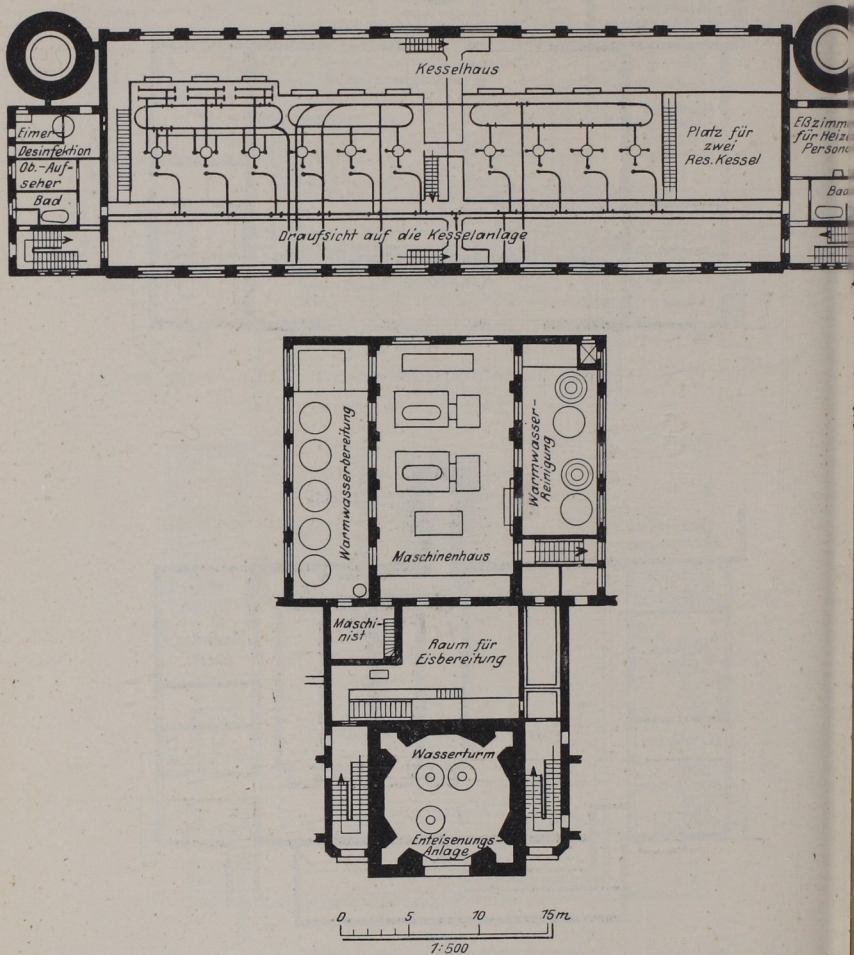
Abb. 201. Hamburg-Barmbeck, städt. Krankenhaus für 2—2400 Betten, Kesselhaus.
