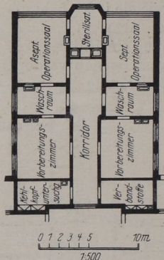
Abb. 149. Delmenhorst, städt. Amtskrankenhaus, Operationsflügel.
