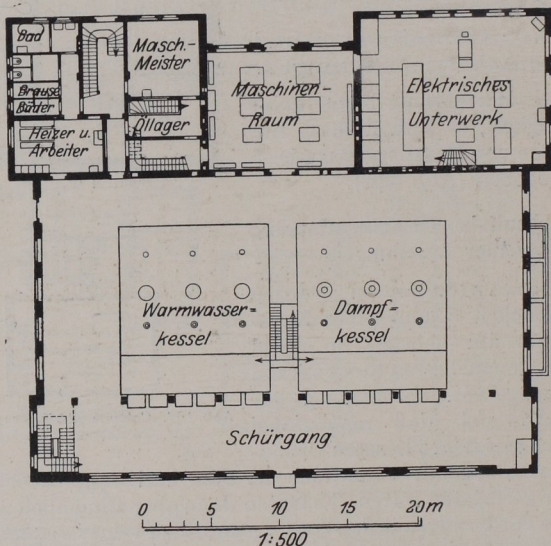
Abb. 200. Leipzig-Eutritsch, städt. Krankenhaus St. Georg für 1920 Betten, Kesselhaus. lauter Einzelhäuser gegeben hat. Aber man blieb mit diesem Grundsatz nicht allein bei den Krankenabteilungen stehen, son-
