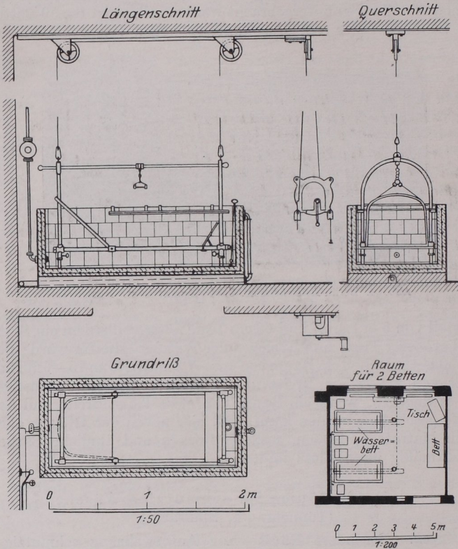
Abb. 35. Hebevorrichtung für Dauerbäder. (Nach RUPPEL.)
