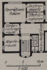
Abb. 147. Operationsabteilung für ein kleines Krankenhaus nach MUSSIGBRODT.
