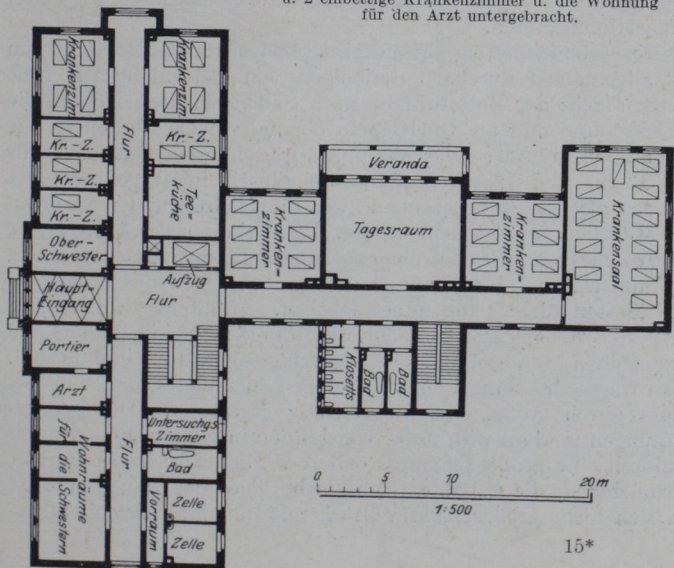
Abb. 209. Lehe a. d. Weser, Krankenhaus f. 150 Betten. Erd- u. Kellerschöß. Das Oberschöß ist ebenso ausgenutzt, wie das Erdschöß, nur in den Räumen der Oberschwester, des Haupteingangs, des Pförtners, des Arztes, u. den Wohnräumen der Schwestern sind 1 Schwester-, 2 zwei- u. 2 einbettige Krankenzimmer u. die Wohnung für den Arzt untergebracht.
