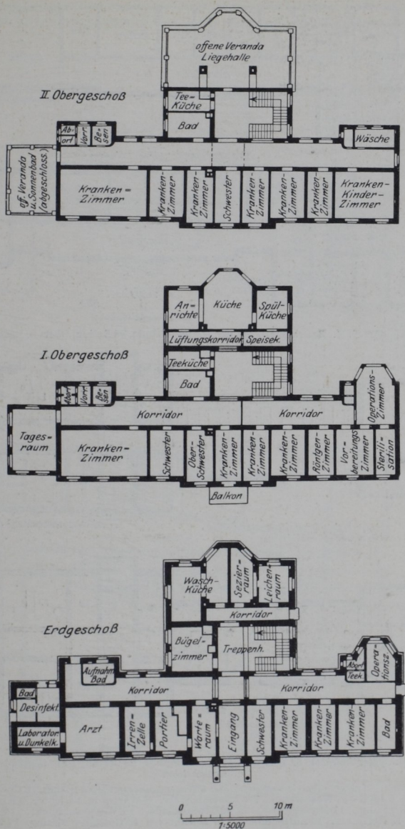
Abb. 204. Kirn, städt. Krankenhaus, 28 Betten, Ober-, Erd- u. Sockelgeschoß.
