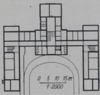
c) Würzburg, Staatliches Luitpold-Krankenhaus. d) Berlin-Reinickendorf, Städtisches Krankenhaus.
