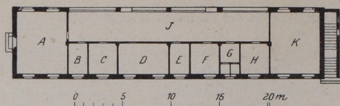
Abb. 129. Düsseldorf, städt. Krankenanstalt, Freiluftabsonderungshaus. A u. K Räume zur Angewöhnung der Kinder und zum Füttern. B Bad. C Wärmküche. D Schwester. E Arztzimmer. F Einzelzimmer. G Abtritte. H Schrank u. Wäschezimmer.
