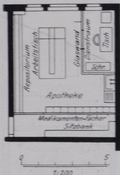
Abb. 86. Dispensierraum einer kleinen Anstalt (nach WOLTJE).
