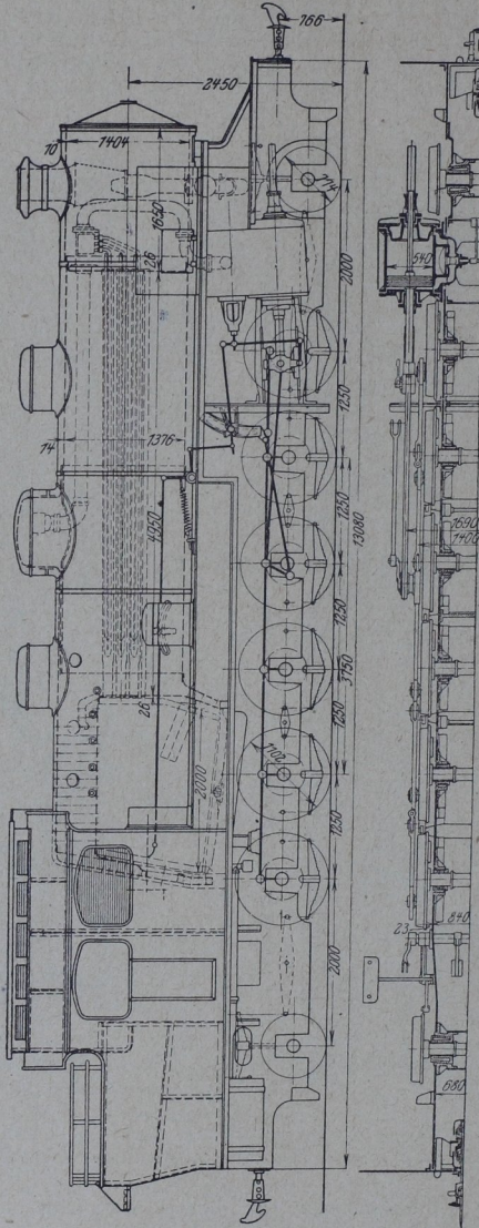
Abb. 532. 1F1-Heißdampf-Zwilling-Tenderlokomotive der holländischen Staatsbahn auf Java.
