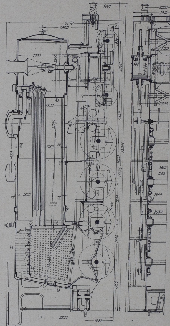
Abb. 483. 2D-Heißdampf-Zwilling-G-Lokomotive der Madrid-Zaragossa-Alicante-Bahn.
