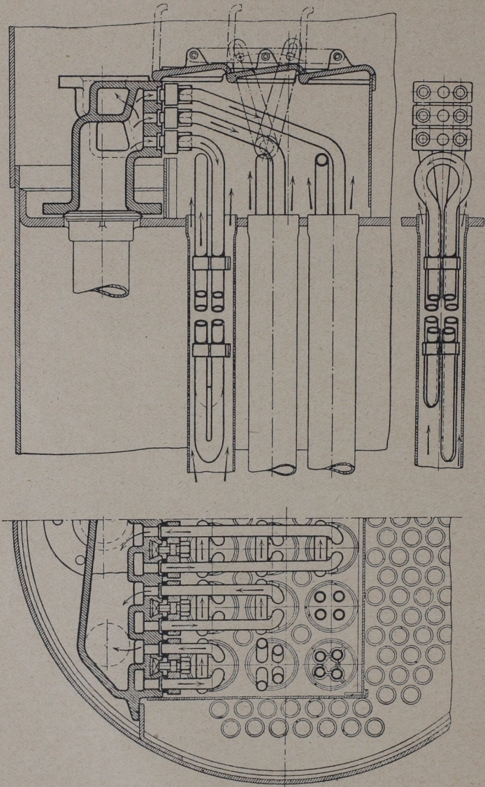
Abb. 141. Großrohrboiler Bauart „Schmidt“ (mit wagerechtem Flansch).
