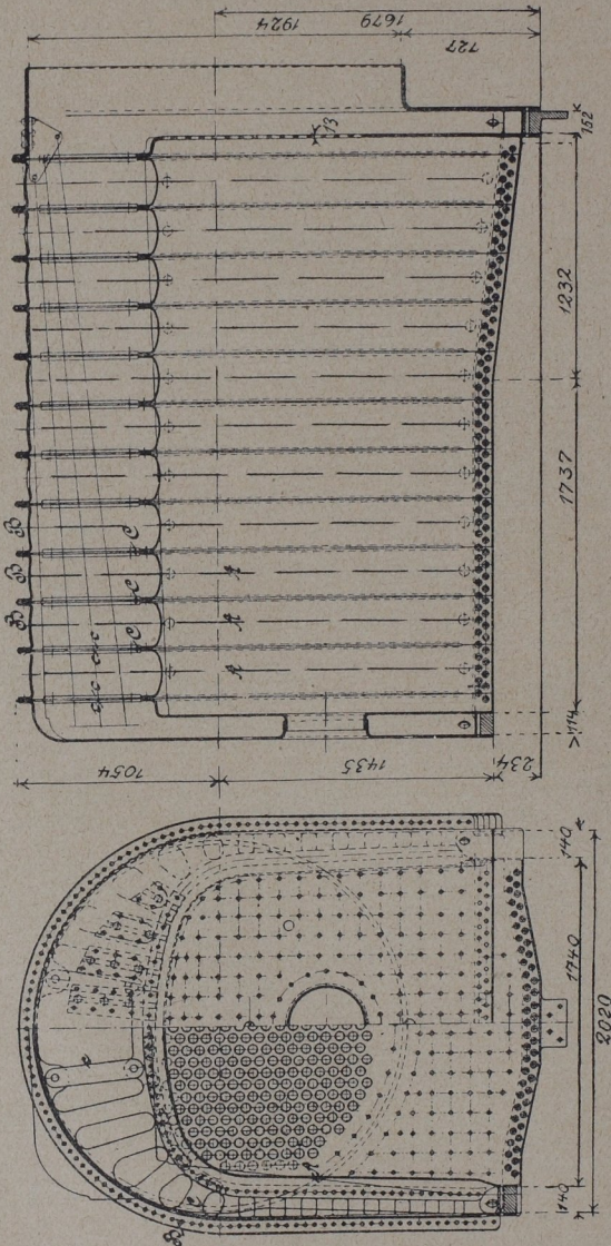
Abb. 95. Jacobs-Shupert-Hinterkessel.
