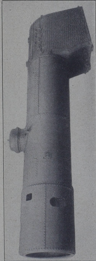
Abb. 88. Kessel der 1C1-Heißdampf-Zwillings-S-Lokomotive für die oldenburgische Staatsbahn (Hanomag).
