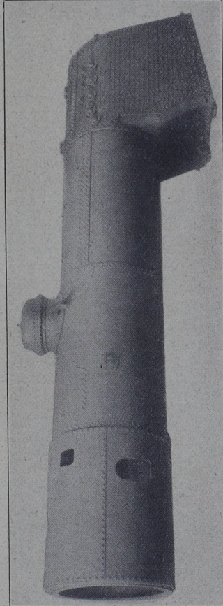
Abb. 88. Kessel der 1CI-Heißdampf-Zwillings-S-Lokomotive für die oldenburgische Staatsbahn (Hanomag).
