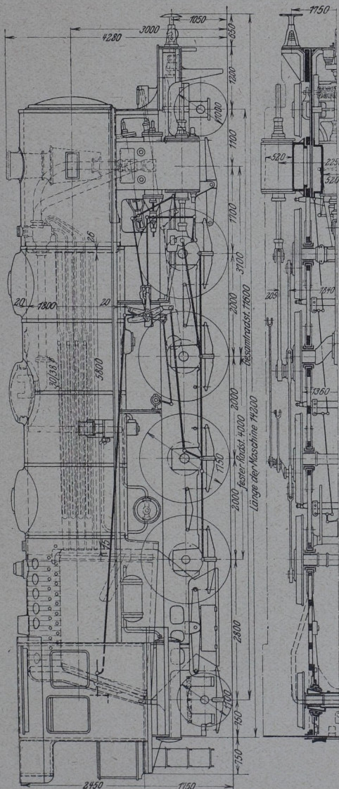
Abb. 404. 1D1-Heißdampf-Drilling-P-Lokomotive Gattung P 10 (Preußen) (Entwurf)
