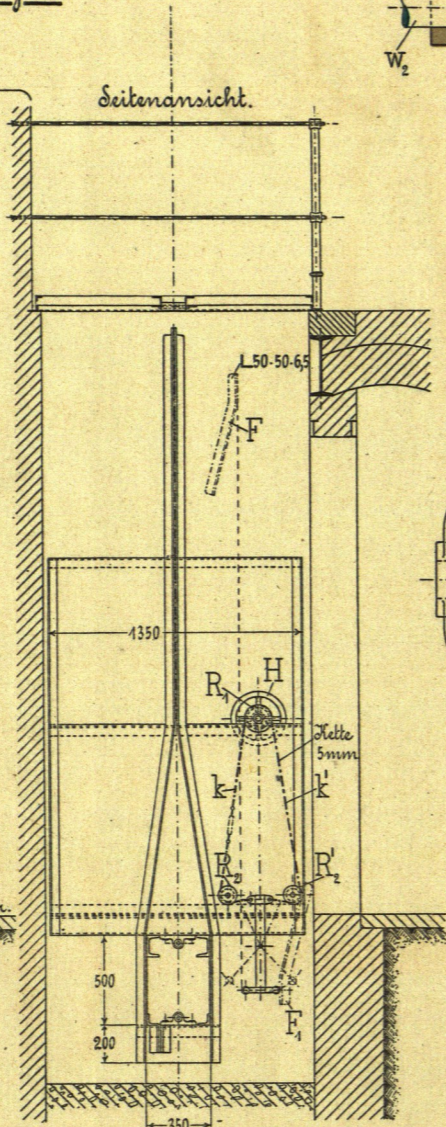
Fig. 1. 1/40.
