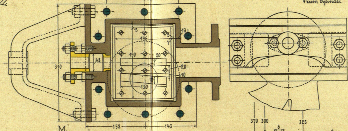
Fig. 3a. 1/2,5.
