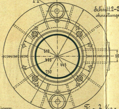
Fig. 3b. 1/2,5.
