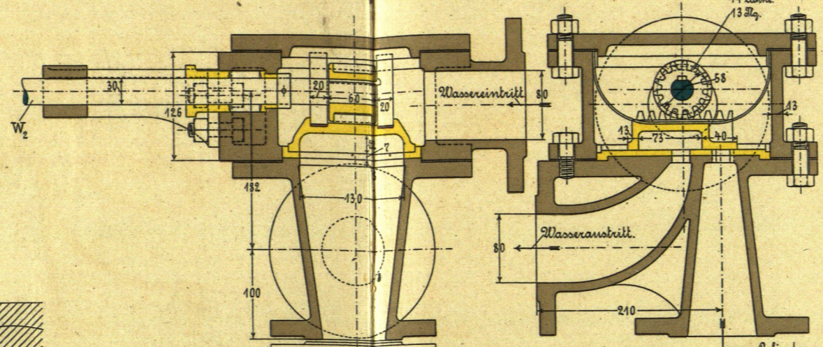
Fig. 2. 1/6. Schieber.
