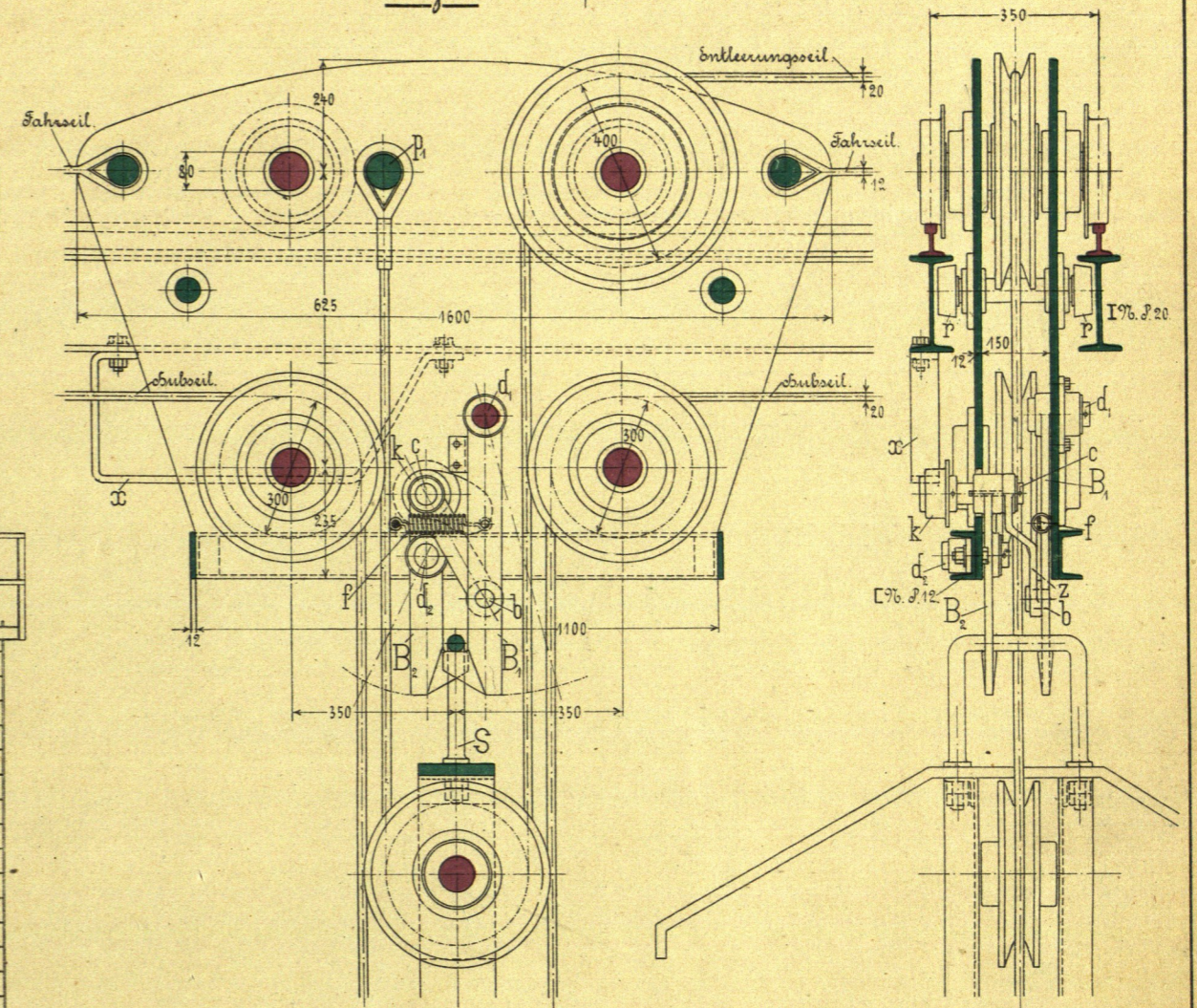
Fig. 2. 1/15. Laufkatze.
